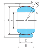
GE...ET-2RS
